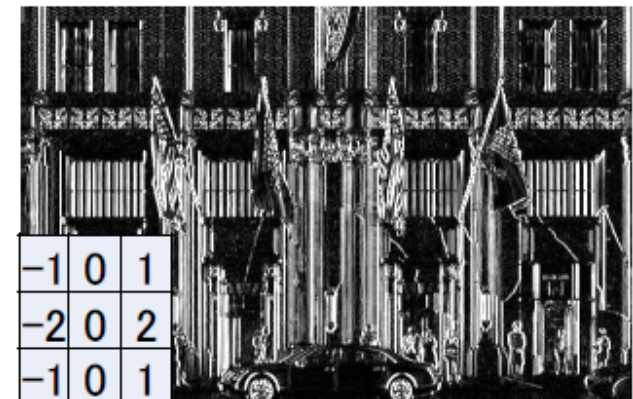
ソーベルフィルタ(横)
